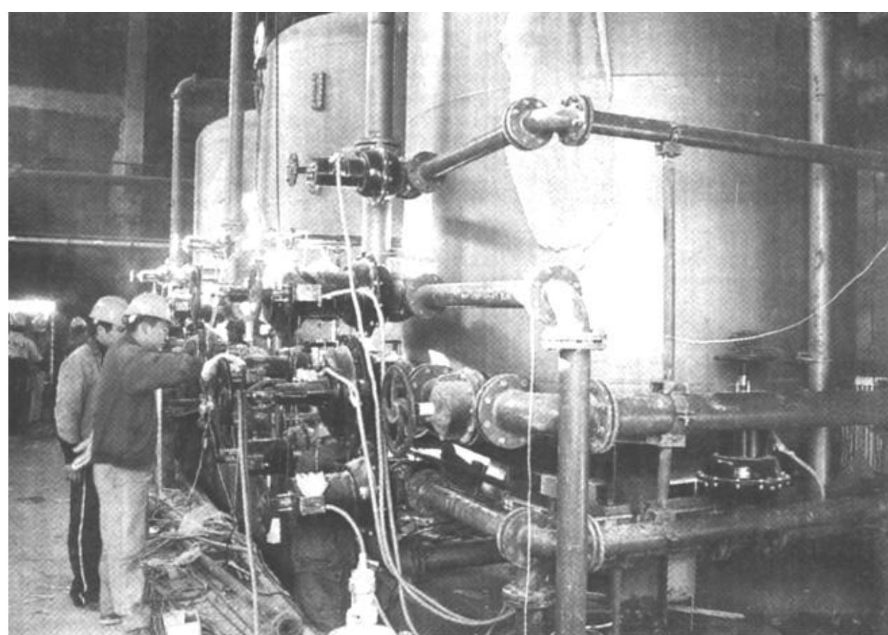
近日，胜利油田基地集中供热工程首站进入收尾调试阶段。为了保证油田基地广大居民冬季取暖，承担施工的胜利油建有限公司二分公司组织青年突击队进行水压调试，以实际行动保证施工质量和工程进度等承诺目标的实现。图为承担调试任务的青工正在检查管线回路阀门的密封性。（刘长青 摄）
